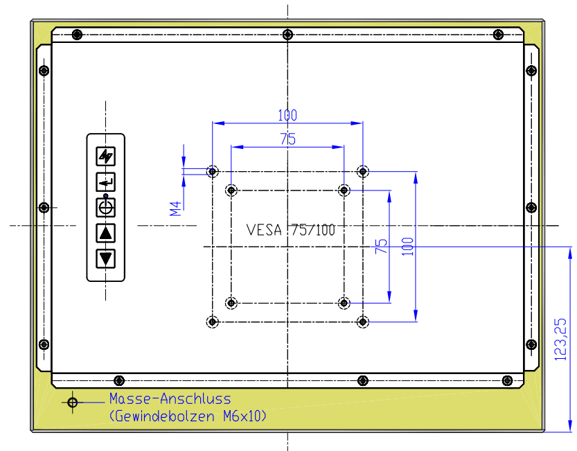
RÜCKANSICHT
