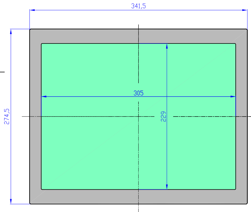
FRONTANSICHT
